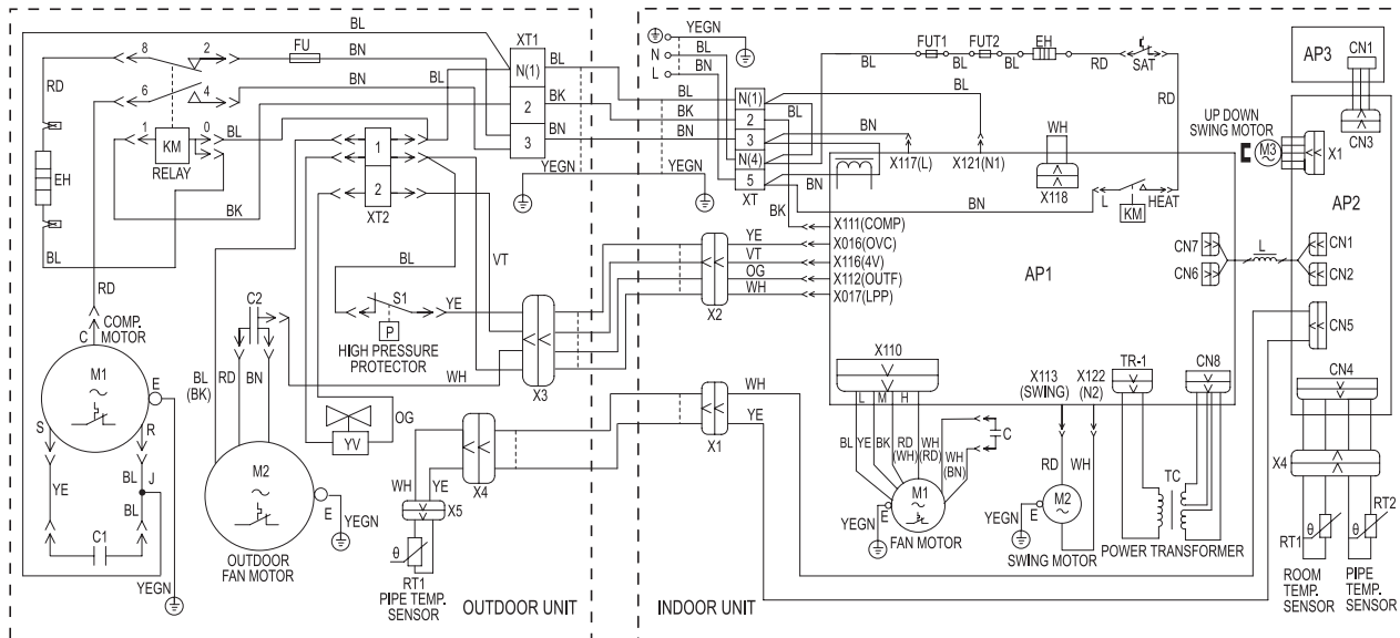
Схема электрическая модели GVHN24A1NK3AA
